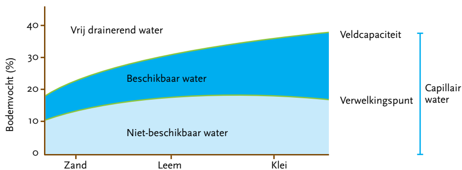
Vochtkarakteristieken van verschillende bodemtypes. (naar Harris)
